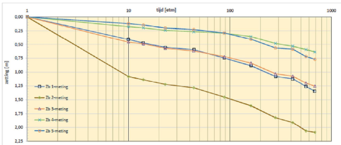
Figuur 3.2: Gemeten zettingen t.p.v. de zakbaken ZB01A t/m ZB5A.
