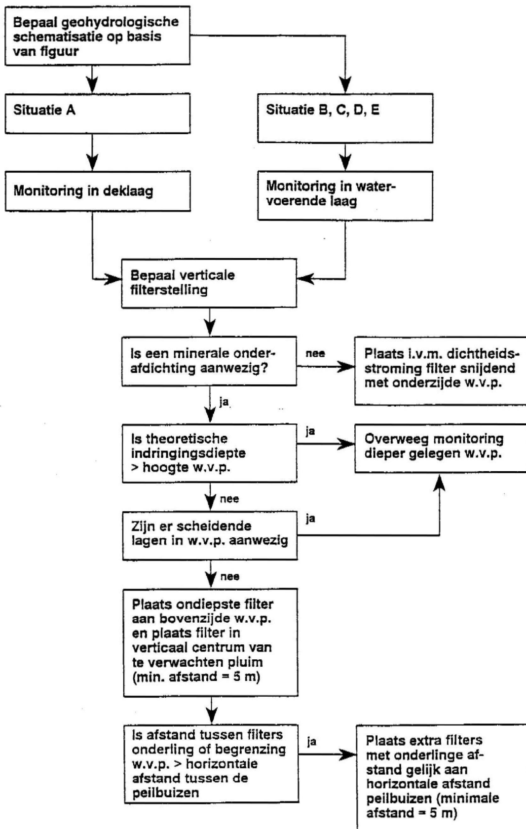
Schema 5 Selectie geohydrologisch systeem en filterstelling
