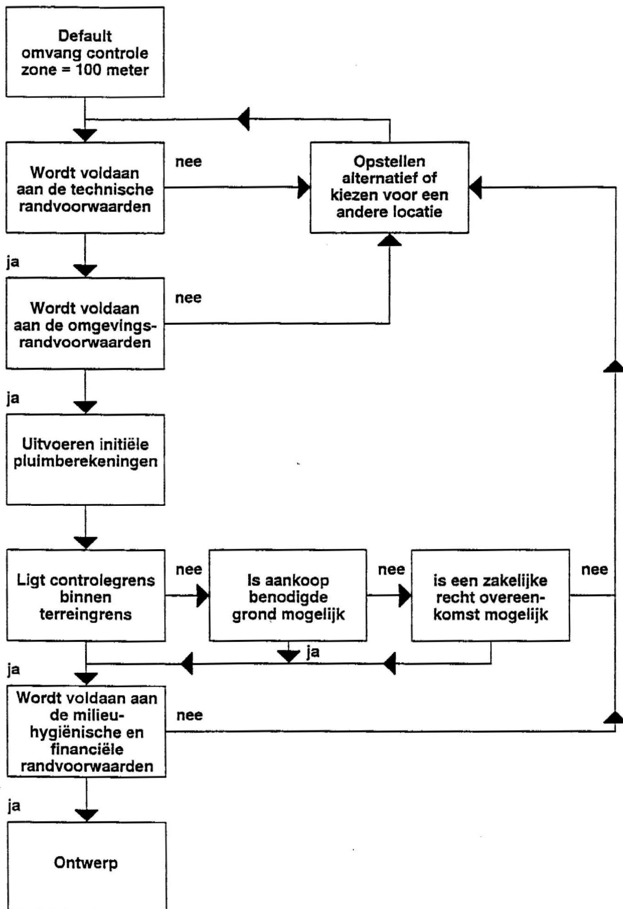
Schema 3 Ontwerpprocedure voor vaststellen omvang controlezone
