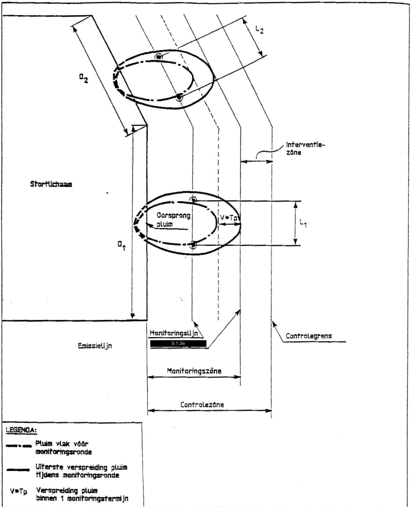
Figuur 1 Zonering en basiselementen monitoringssysteem
