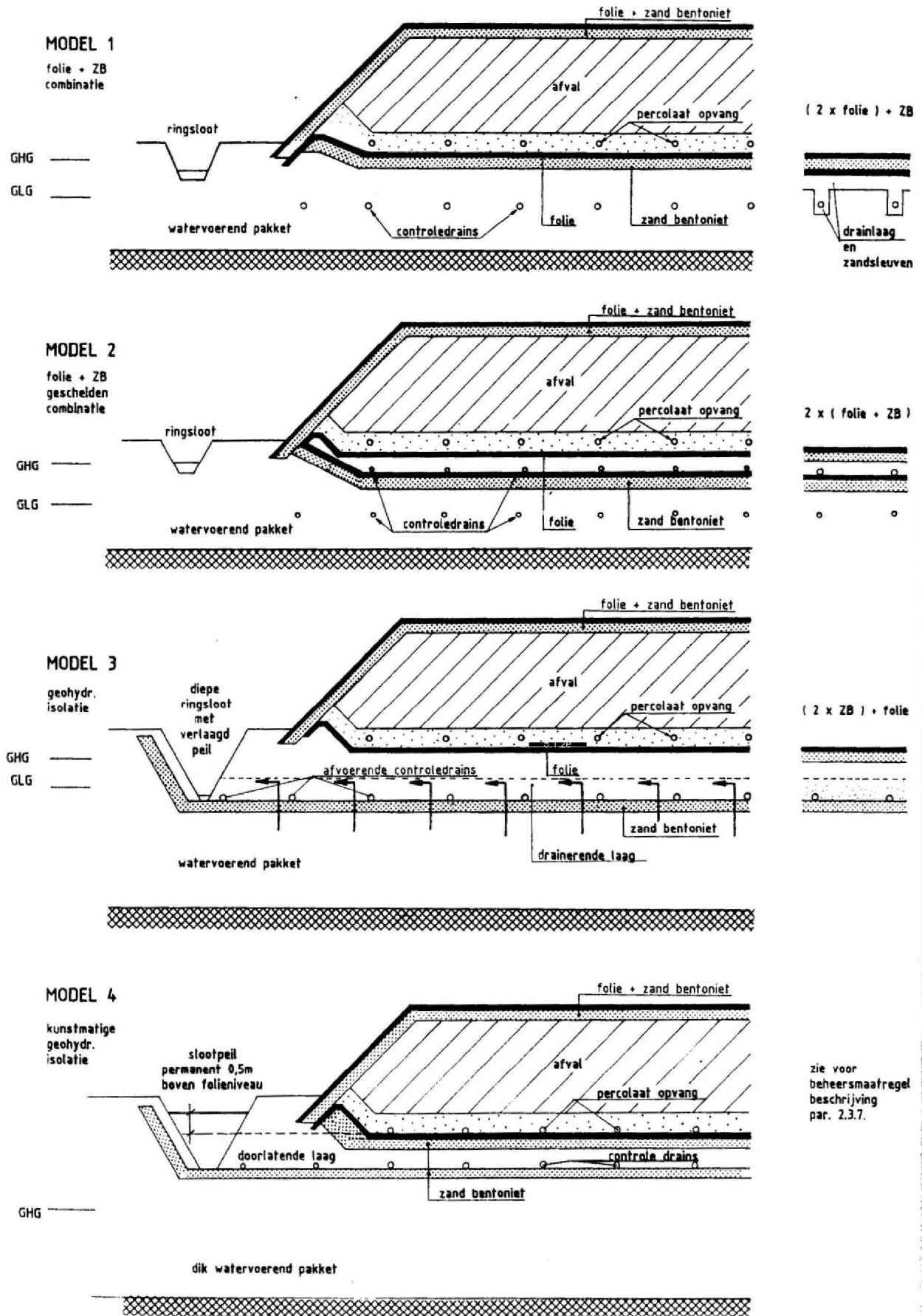
figuur 4 Onderafdichtingsconstructies
