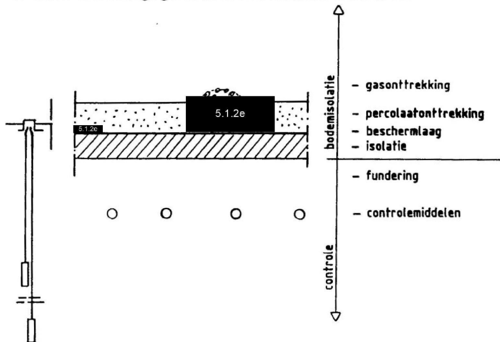
Figuur 1: Opbouw referentie-onderafdichting
