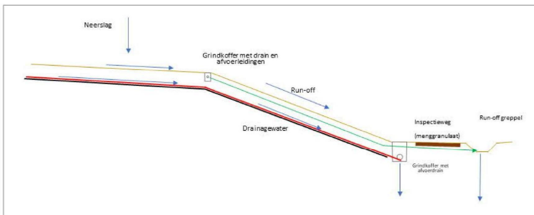
Figuur 3-5: Hemelwaterafvoer talud zuidoost zijde 1° ontwerpfase (schematisch)
