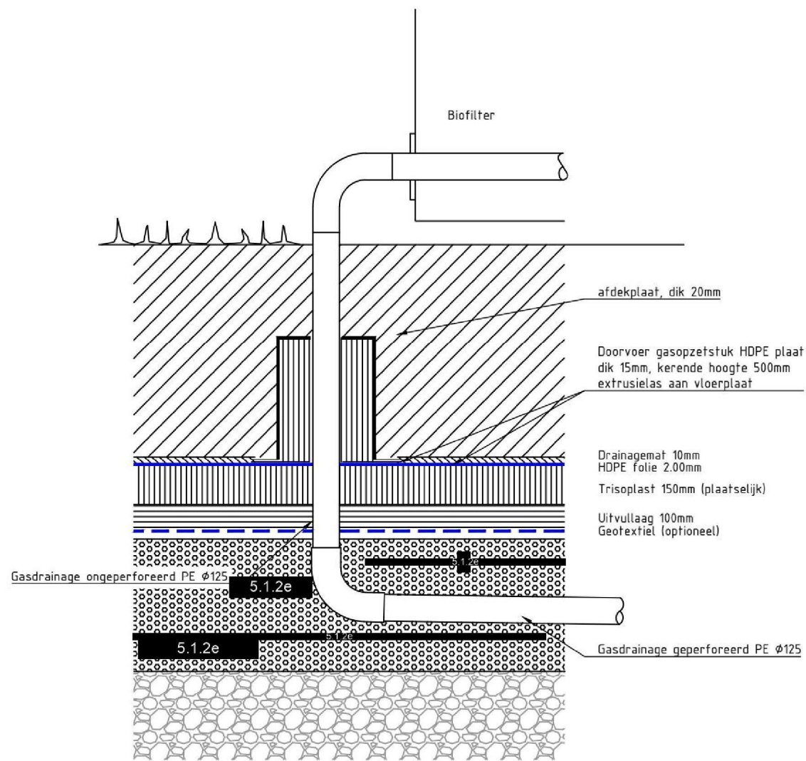
Detail doorvoer gasdrainage Schaal 1:20
