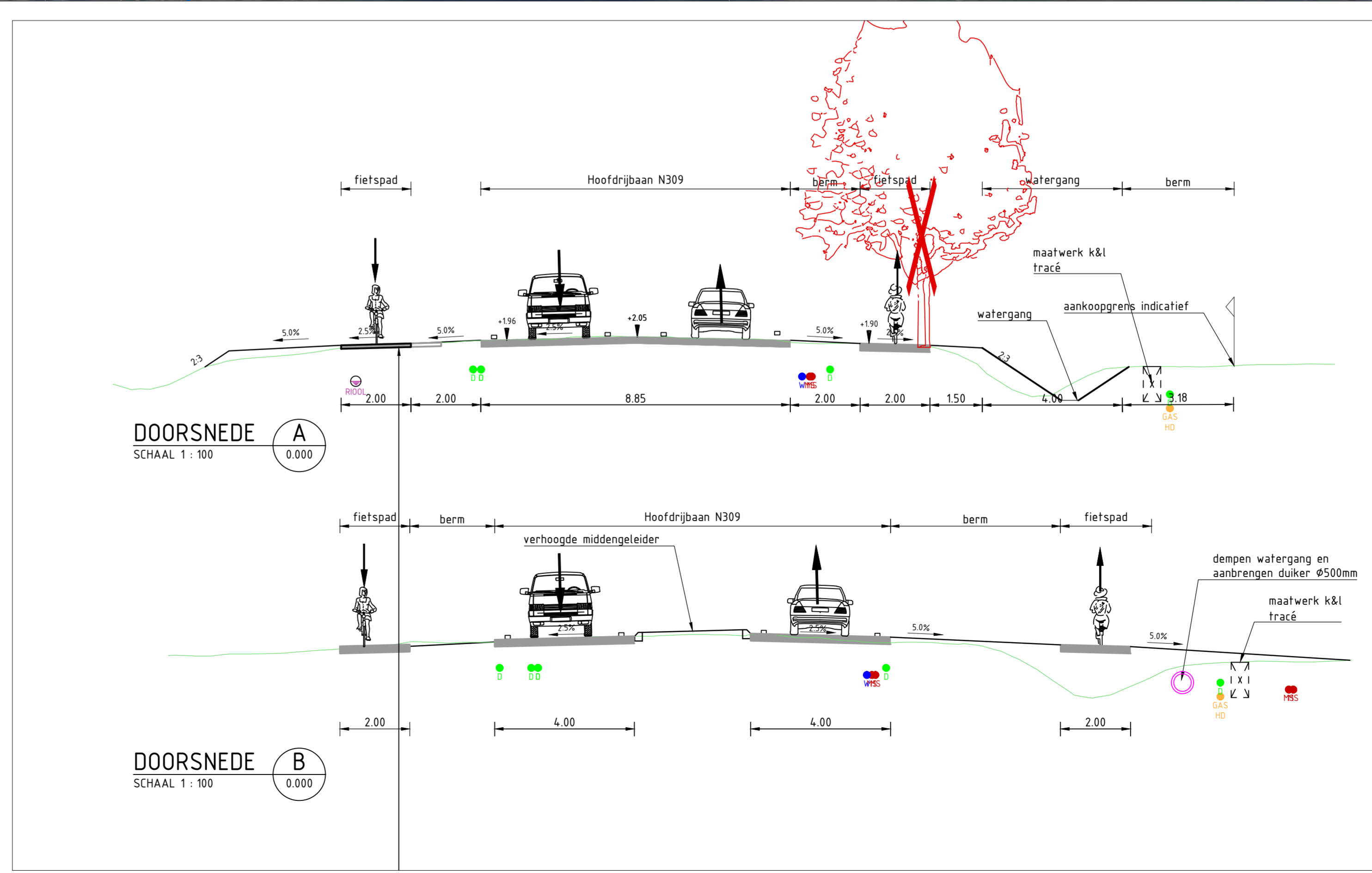
N309 Zuiderzeestraatweg oost: Rechts in en rechts uit met middengeleider t.b.v. (brom)fiets-oversteek Stoopschaarweg
