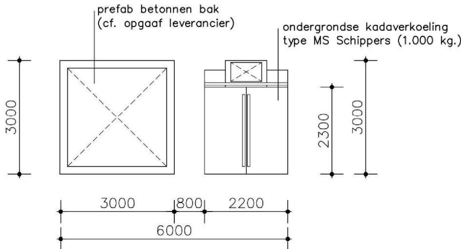
plattegrond opstelling kadaverkoeling
