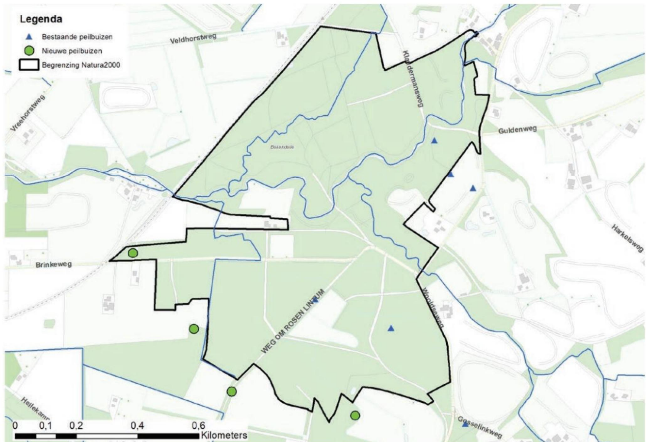
Ontwerp meetnet Peilbuizen Bekendelle
