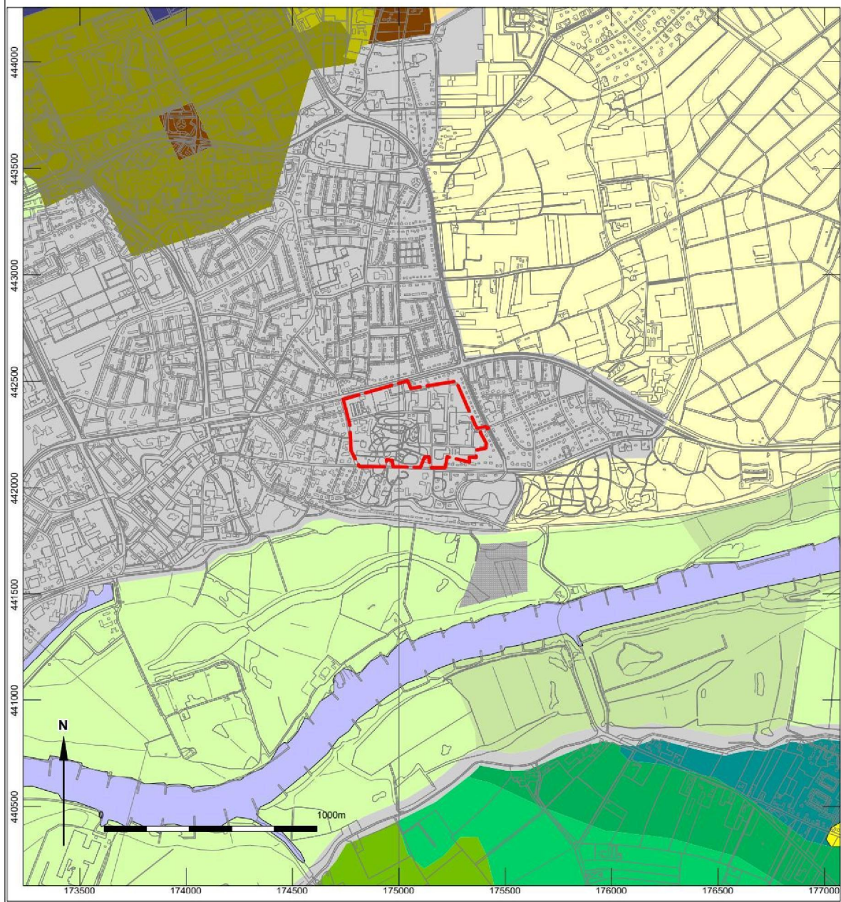
AFBEELDING 3 BODEMKAART
