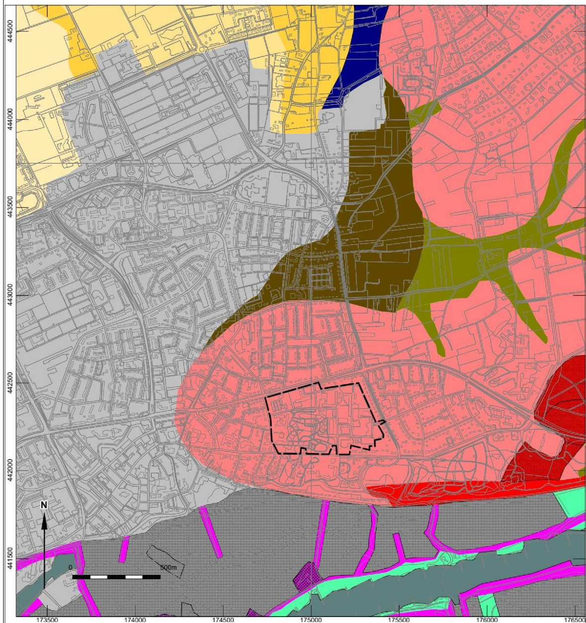
AFBEELDING 2 GEOMORFOLOGIE
