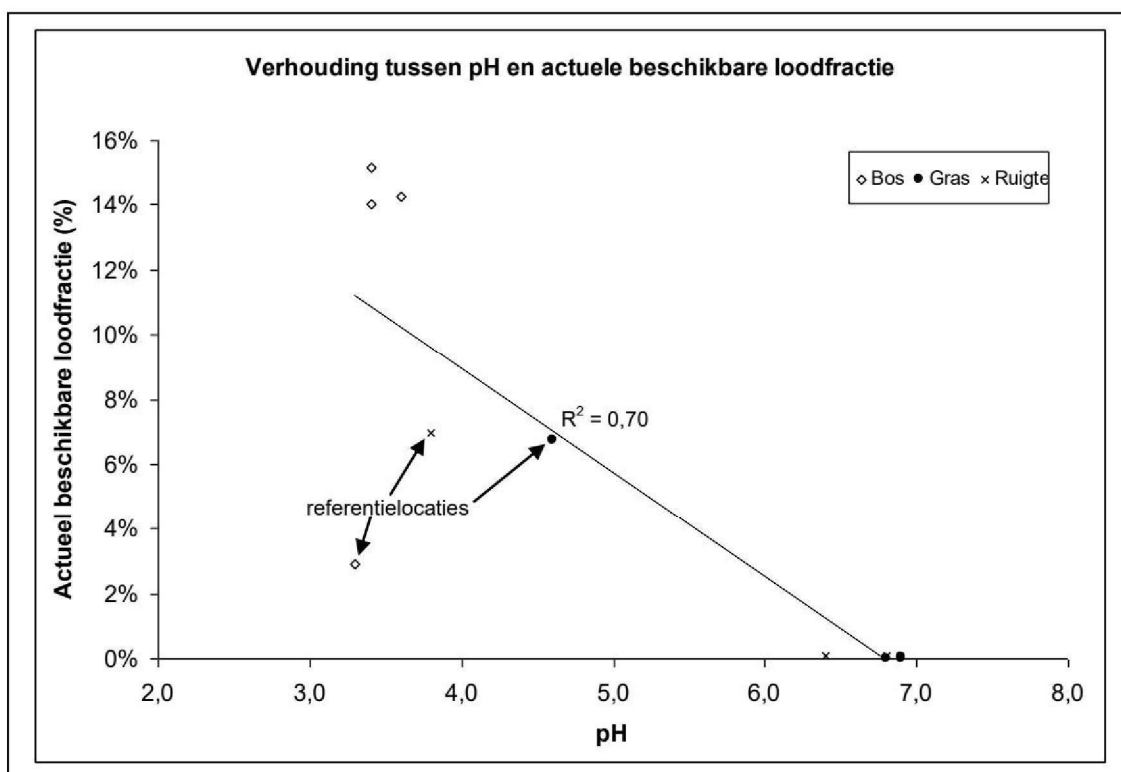
Figuur 3.3 - Verhouding tussen pH en actueel beschikbare loodfractie (actueel beschikbaar gehalte / potentieel beschikbaar gehalte). Bij een oplopende pH neemt de actuele beschikbaarheid af. De lage pH zorgt voor een grotere beschikbare fractie op de boslocaties dan op de gras- en ruigtelocaties met een hoge pH. Er is een redelijke trend waarneembaar met een R^2_{\text{lineair}} van 0,70.
