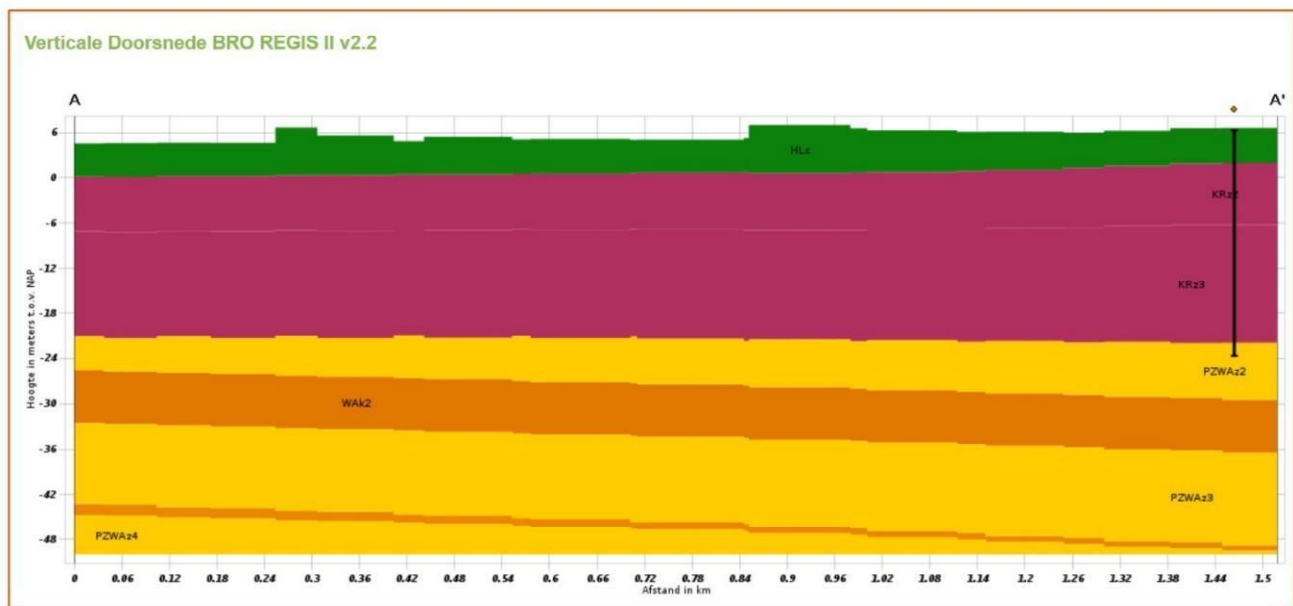
Figuur 1: REGIS doorsnede. HLc = Holocene Complex; KRz2 en 3 = tweede en derde zandige eenheid van de Formatie van Kreftenheye; PZWAz2, 3 en 4: tweede, derde en vierde zandige eenheden van de Formatie van Peize en Waalre; WAK2 = tweede kleiige eenheid van de Formatie van Waalre. Tussen PZWAz3 en PZWAz4 komt nog een dunne derde kleiige eenheid van de Formatie van Waalre voor.
