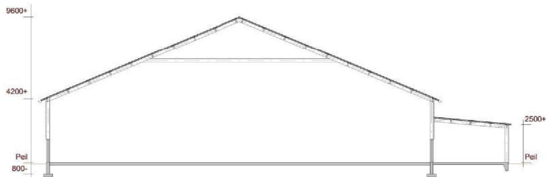
Doorsnede B-B
