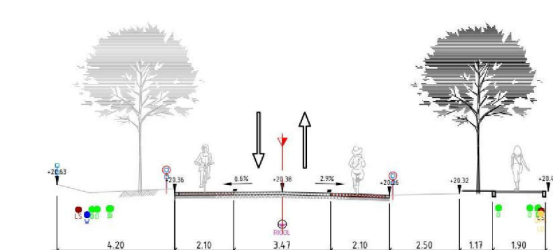
DOORSNEDE 13 SCHAAL 1 : 100
