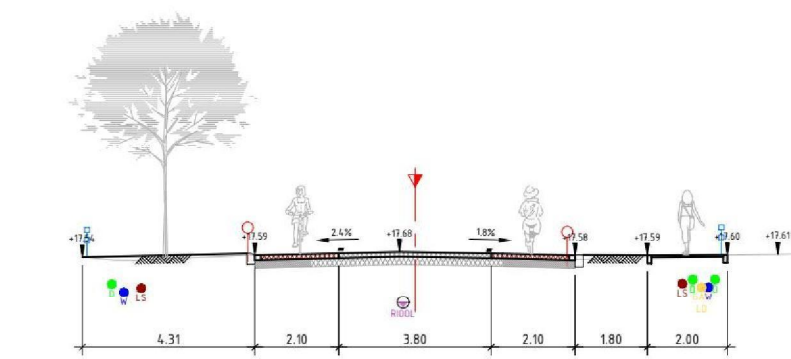
DOORSNEDE 15 SCHAAL 1 : 100
