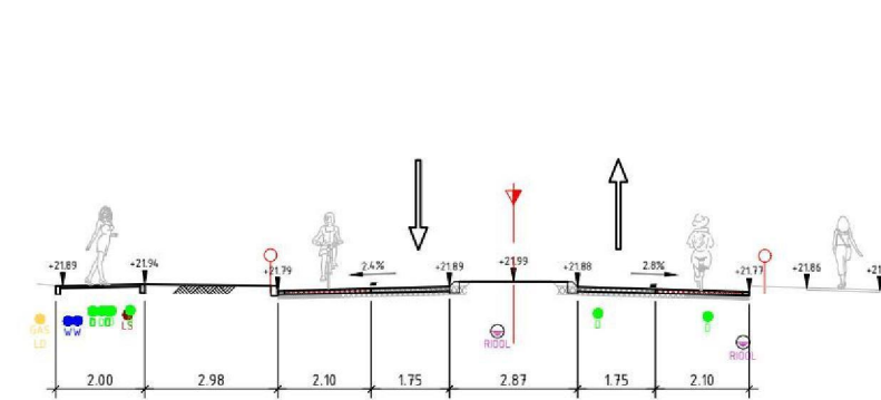
DOORSNEDE 11 SCHAAL 1 : 100
