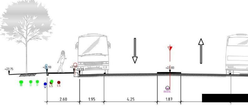
DOORSNEDE 5 SCHAAL 1 : 100
