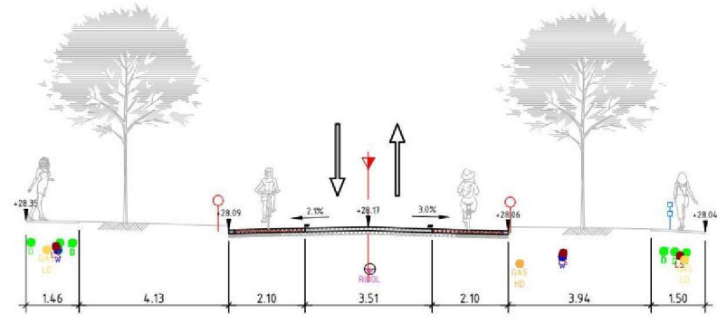
DOORSNEDE 3 SCHAAL 1 : 100
