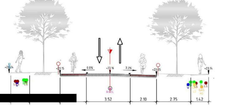
DOORSNEDE 10 SCHAAL 1 : 100
