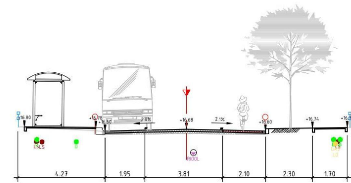
DOORSNEDE 16 SCHAAL 1 : 100
