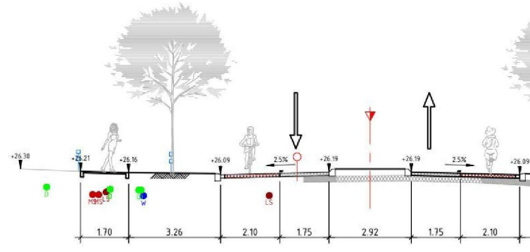
DOORSNEDE 8 SCHAAL 1 : 100
