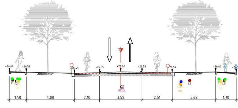
DOORSNEDE 4 SCHAAL 1 : 100
