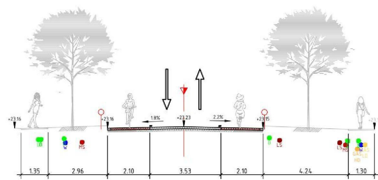
DOORSNEDE 6 SCHAAL 1 : 100
