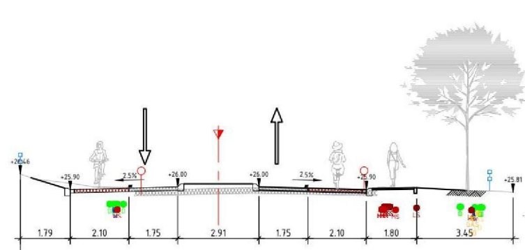
DOORSNEDE 7 SCHAAL 1 : 100
