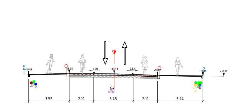
DOORSNEDE 14 SCHAAL 1 : 100
