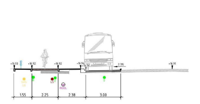
DOORSNEDE 17 SCHAAL 1 : 100
