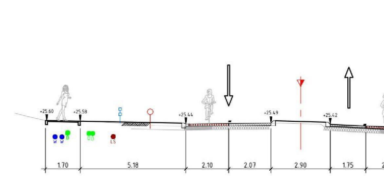
DOORSNEDE 9 SCHAAL 1 : 100
