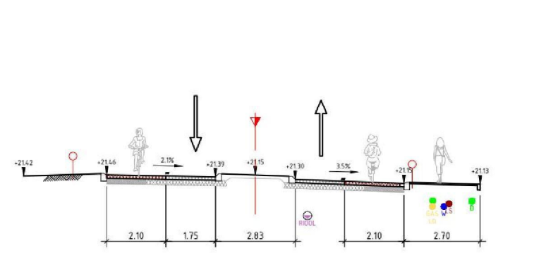
DOORSNEDE 12 SCHAAL 1 : 100
